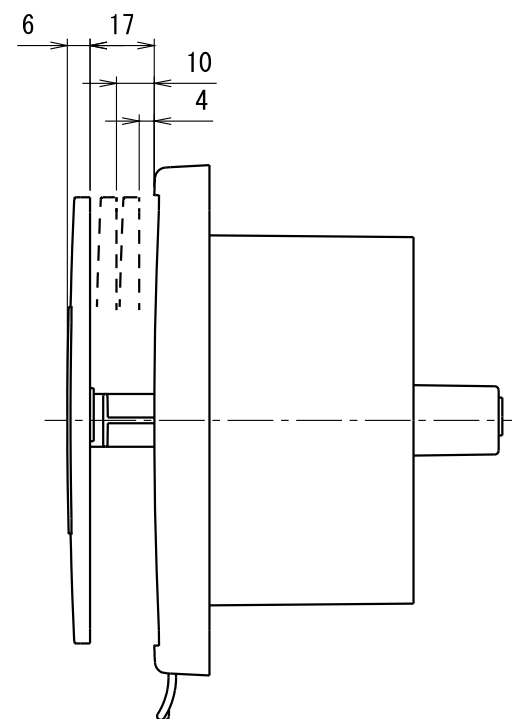
開閉動作図
